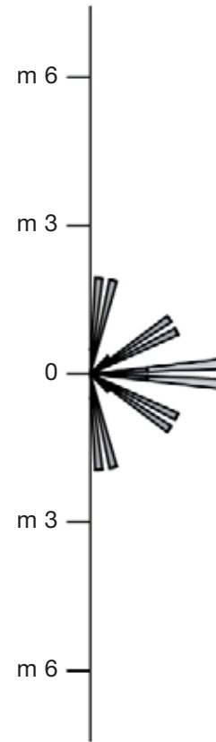
Vista laterale (zona antistrisciamento)
