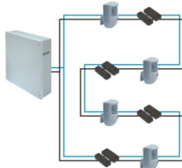
Linea multiplexer con loop chiuso consigliata per LUNGHE DISTANZE
