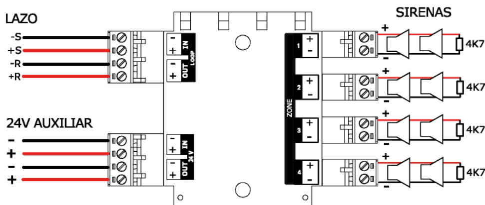
Fig. 27 Dettaglio del cablaggio del modulo analogico delle uscite monitorate
