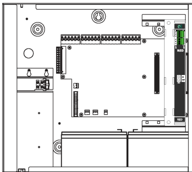
Figura 31 Dettaglio della posizione della scheda di rete FA-MNW-EV.
