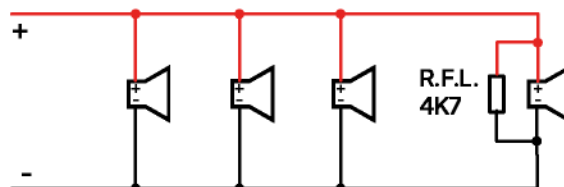
Figura 26 Cablaggio polarizzato della sirena
