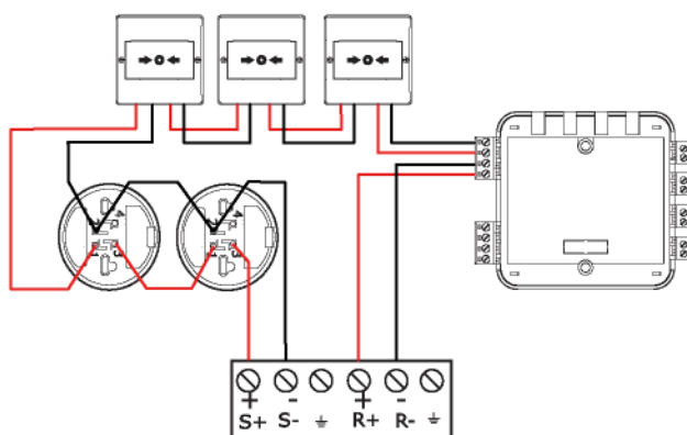
Figura 16 Esempio di collegamento ad anello analogico
