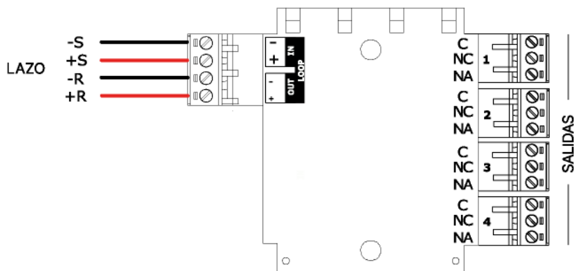
Figura 23 Dettaglio del cablaggio del modulo di uscita analogica
