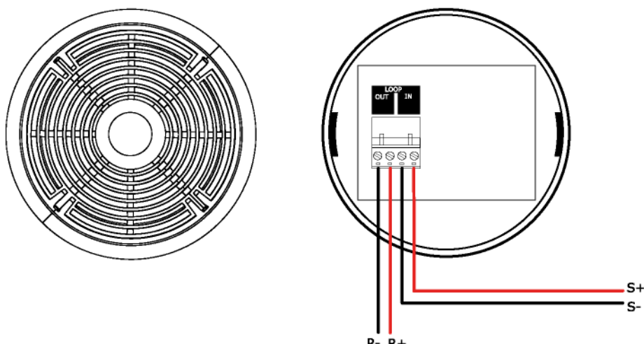
Figura 21 Dettaglio del cablaggio di una sirena analogica
