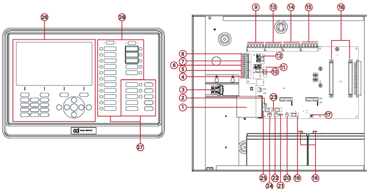
Figura 2 Elementi della centrale elettrica FA-Cxx25-EV
