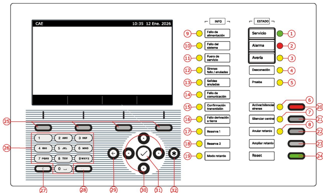
Figura 39 Parte anteriore centrale CAE-300
