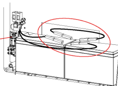
Figura 12 Collegamento della batteria
