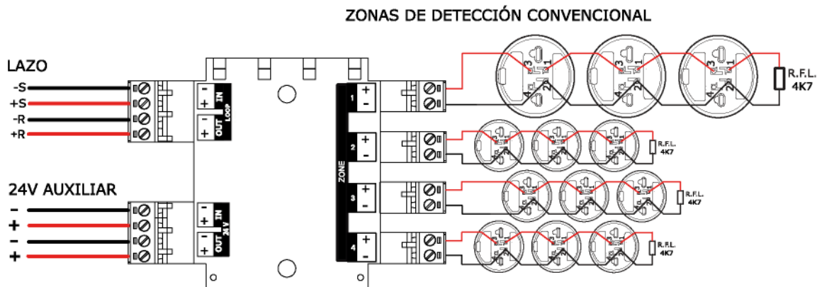
Fig. 28 Dettaglio del collegamento del modulo analogico delle zone convenzionali
