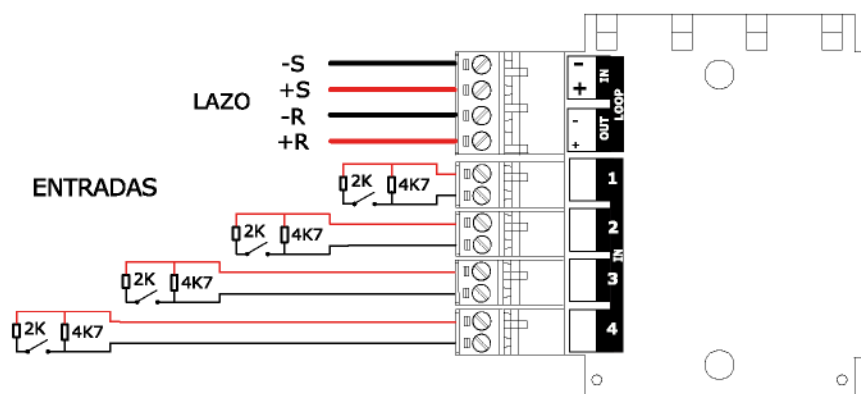
Figura 22 Dettaglio del cablaggio del modulo di ingresso analogico
