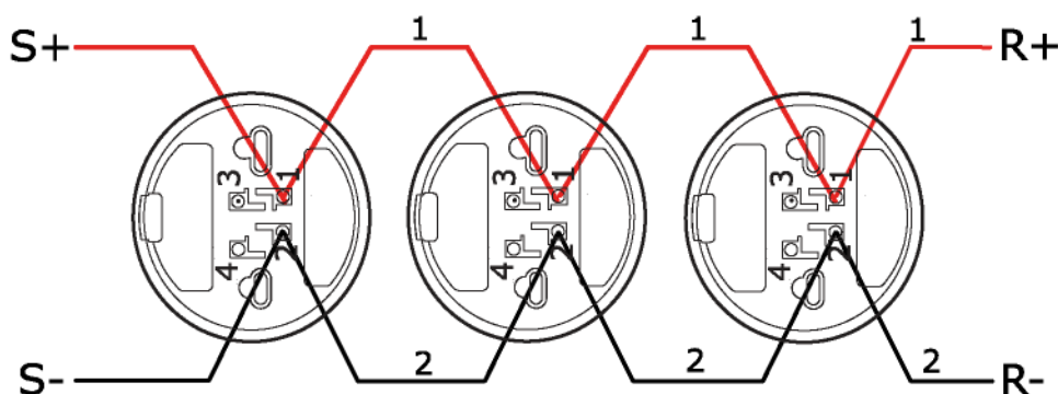
Figura 18 Collegamento di un circuito analogico con rivelatori senza isolatore
