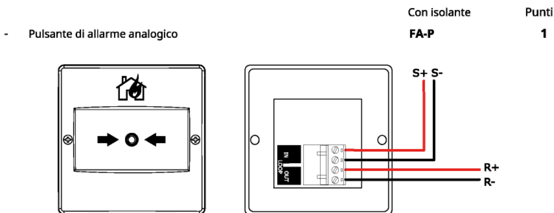
Figura 20 Dettaglio del cablaggio di un pulsante di allarme analogico
