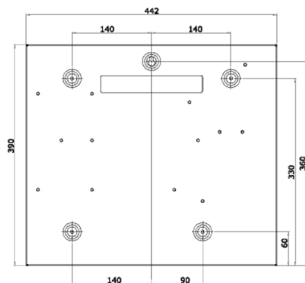
Figura 6 Dimensioni per il montaggio della scatola a parete
