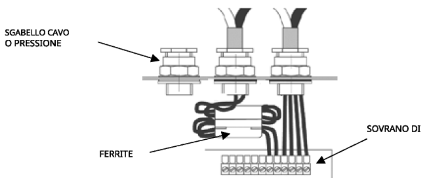
Figura 9 Esempio di collegamento, utilizzando pressacavi e ferrite
