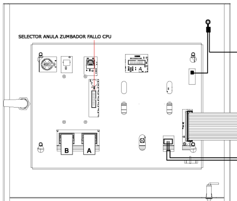
Figura 29 Posizione del selettore di override del cicalino in caso di guasto del sistema
