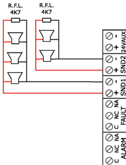
Figura 4 Terminali di connessione Uscite centrali FA-Cxx25-EV
