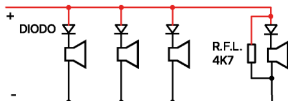
Figura 25 Cablaggio delle sirene non polarizzate
