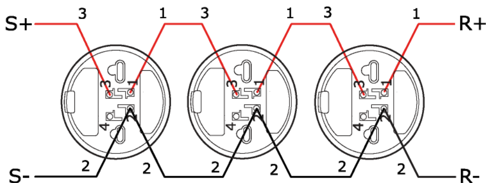
Figura 17 Collegamento di un circuito analogico con rivelatori a isolatore
