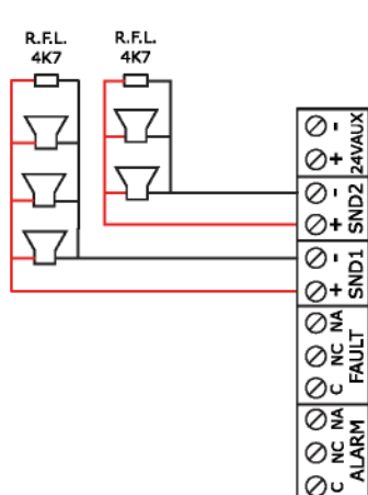
Figura 14 Cablaggio dell'uscita della sirena
