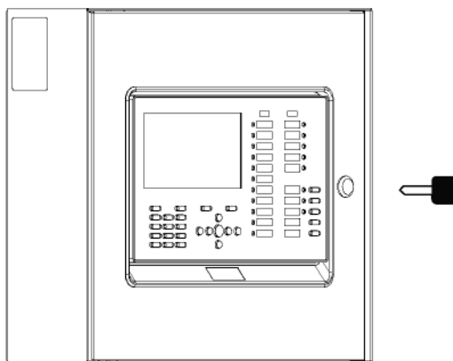
Fig. 5 Per aprire l'unità di controllo FA-Cxx25-EV utilizzare la chiave della serratura della porta
