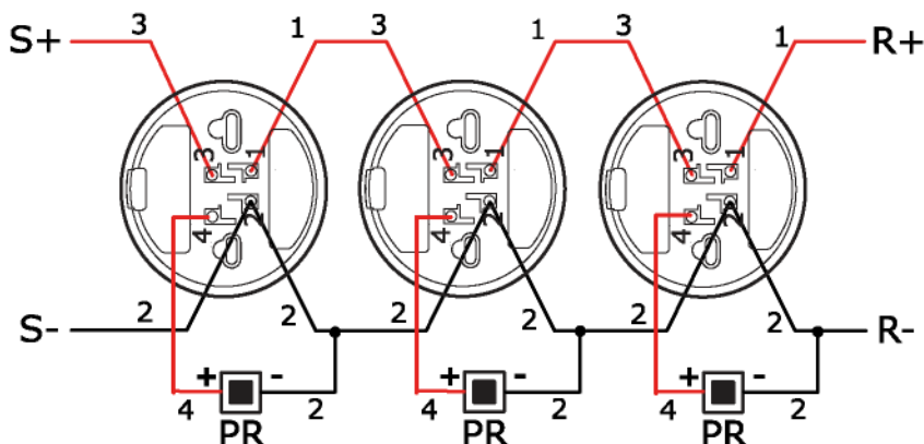
Figura 19 Collegamento dei rilevatori con la spia luminosa di indicazione dell'azione
