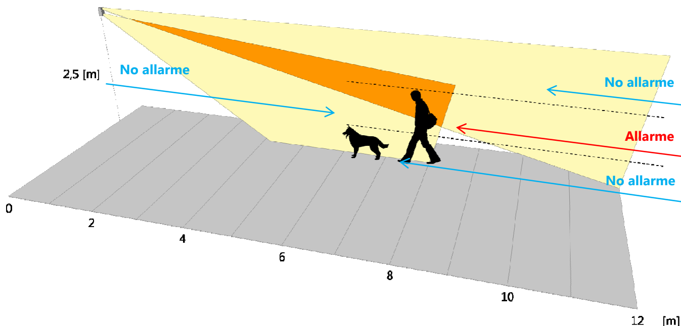
Fig. 4 - Funzionamento in AND: l'uomo genera allarme, il cane no
