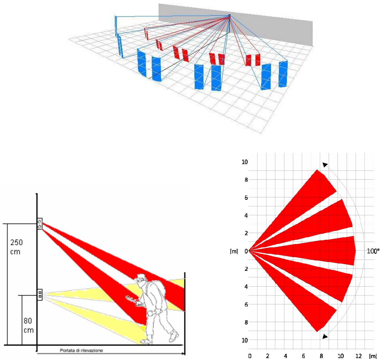
Fig. 1 - Disposizione dei fasci delle testine ad infrarosso
